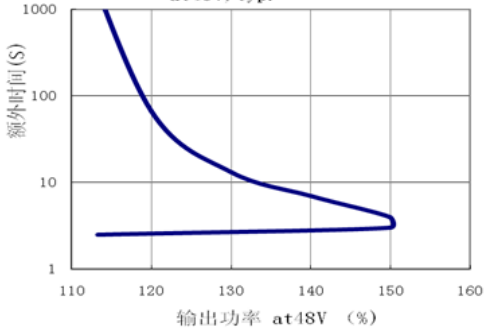
图 3-5-2 额外时间VS输出功率 at48V, typ.
