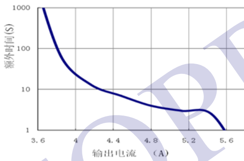
图 3-6-1 额外时间VS输出电流, typ.
