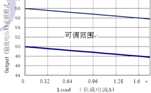
图 3-2-2 Output V-I curve 并联模式 (输出负载特性曲线)
