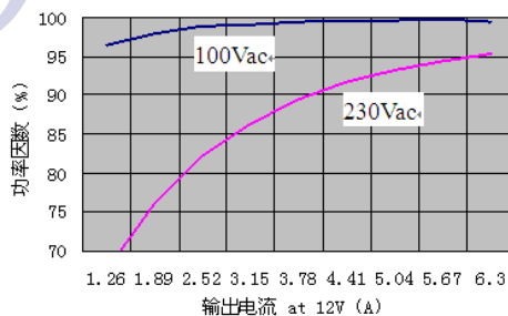
图1-4 功率因数VS输出电流 at 12V, typ
