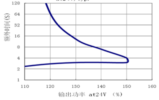
图 3-5-1 额外时间VS输出功率 at24V, typ.
