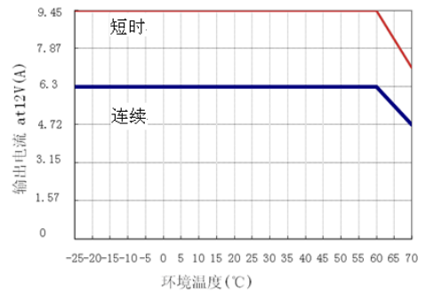
图6-1 输出电流VS环境温度 at12V, typ.
