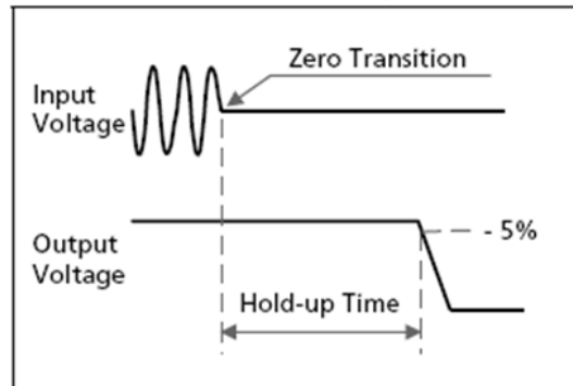
图 3-4 关机曲线
