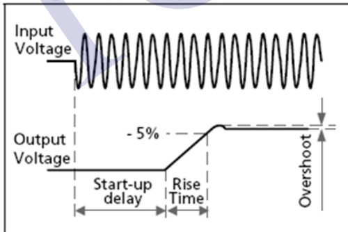
图 3-3 开机曲线
